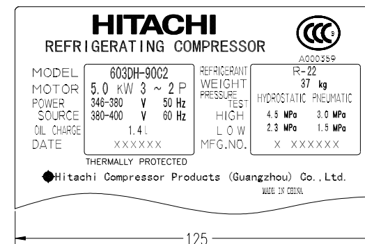
铭牌 Name Plate
