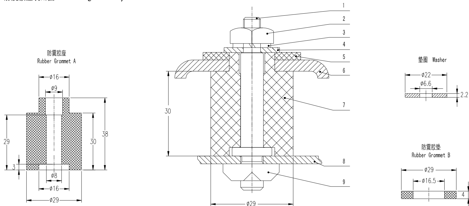
支撑螺栓 Bolt
