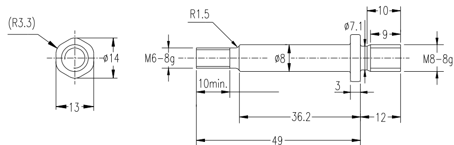
支撑螺栓 Bolt
